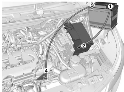
Séquence de raccordement des câbles :
